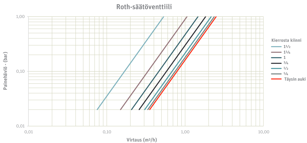
Roth-säätöventtiilin painehäviökäyrät, täysin auki-asennosta 1 1/2 kierrosta kiinni-asettoon
