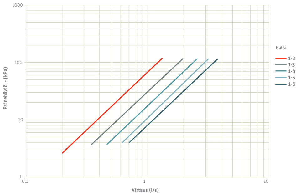
Roth-jakotukkijärjestelmän painehäviökäyrät, 2-3-4-5-6 piiriä auki
