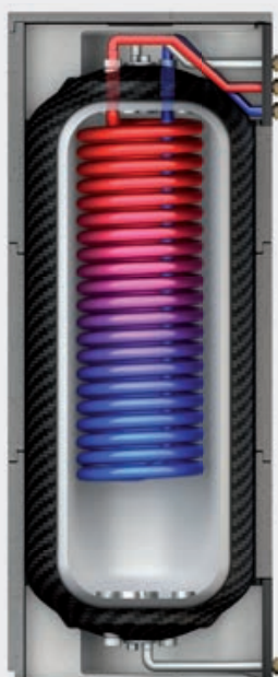
■ Käyttövesivaraaja TQ-TW 325 l / 500 l / 850 l
