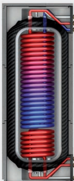
■ TQ-TWS Käyttövesivaraaja lisälämpökierukalla 325 l / 500 l / 850 l
